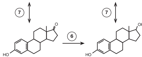
Estrone
