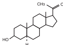
Iso-allopregnanolone
