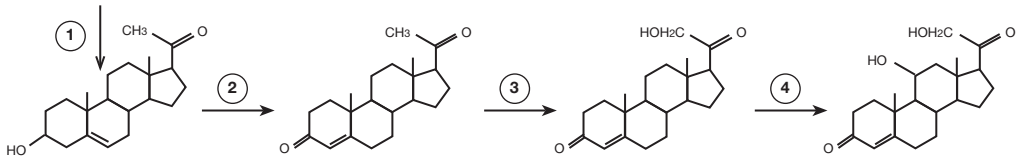
Pregnenolone
