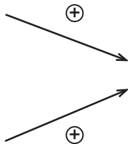
Progesterone
